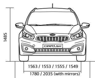
cee'd Sportswagon – exteriöra dimensioner (mm)
