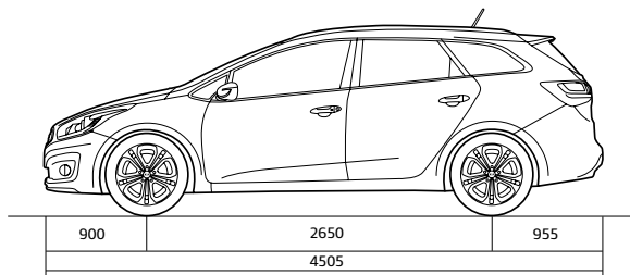
cee'd Sportswagon – exteriöra dimensioner (mm)
